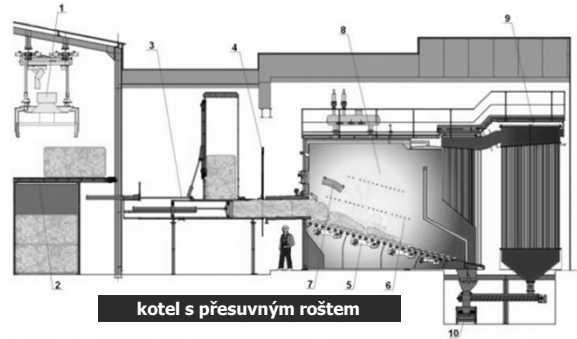
Roštový kotel na slámu 1 - 5 MW
