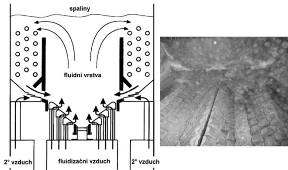
Fluidní rošt s bublinkující fluidní vrstvou
