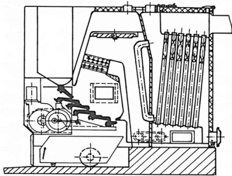
Kotel s přesuvným roštem o výkonu 200 kW
