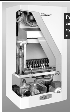
spalinový výměník
